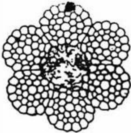
Рис. 7. Уменьшение площади поперечного сечения проволок (интенсивная внутренняя коррозия)
